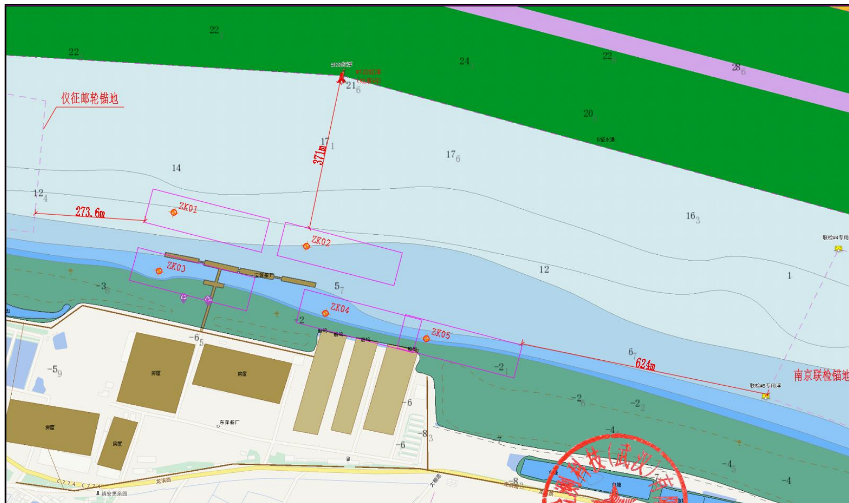
图 2 施工水域与周边水工设施位置关系图示意图
