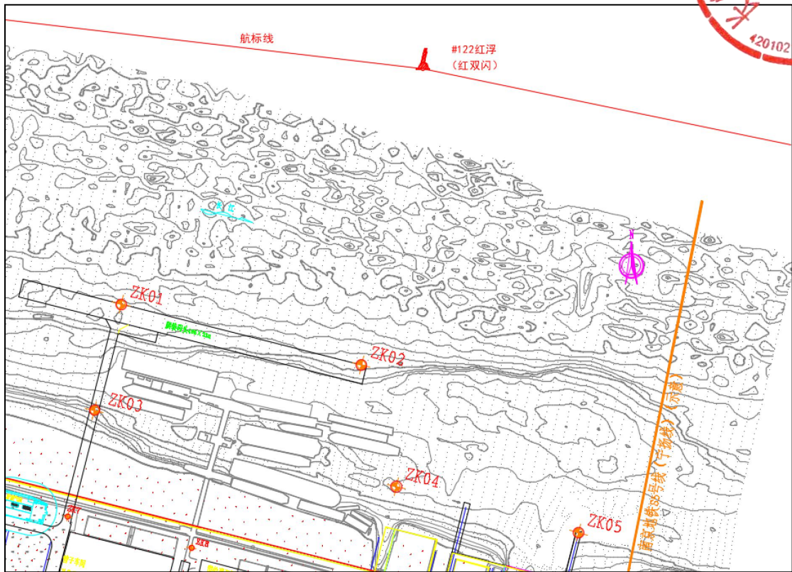
图 2 勘察区水域钻孔平面布置示意图
